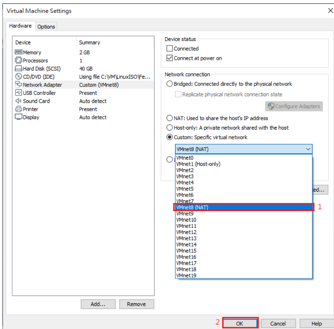
Figure 22 選擇 VMnet (NAT)
